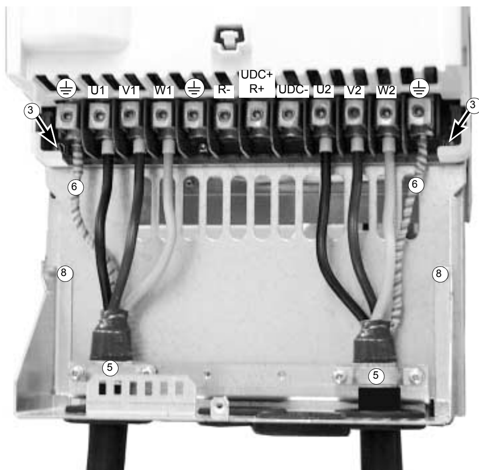
Шасси типоразмера R5
